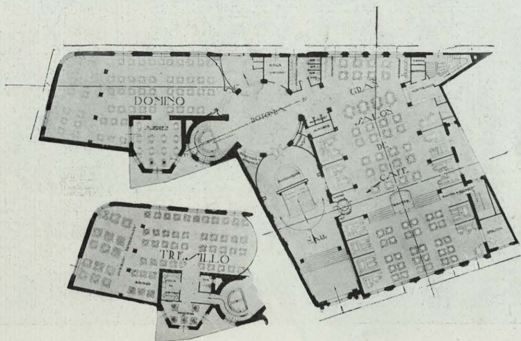
PIANTA DE ENTRESUELO.
