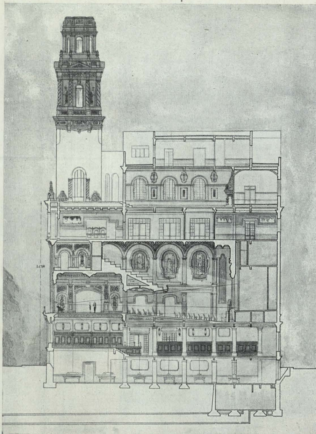
SECCIÓN.
